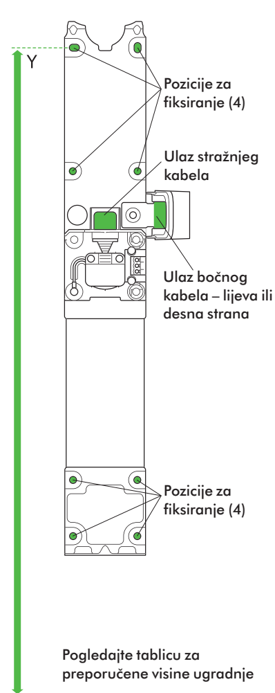
Stražnja ploča
