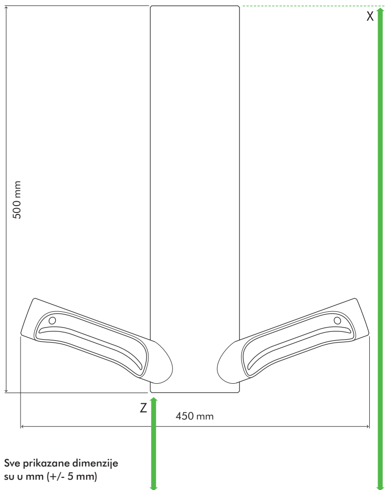
Prednji prikaz
