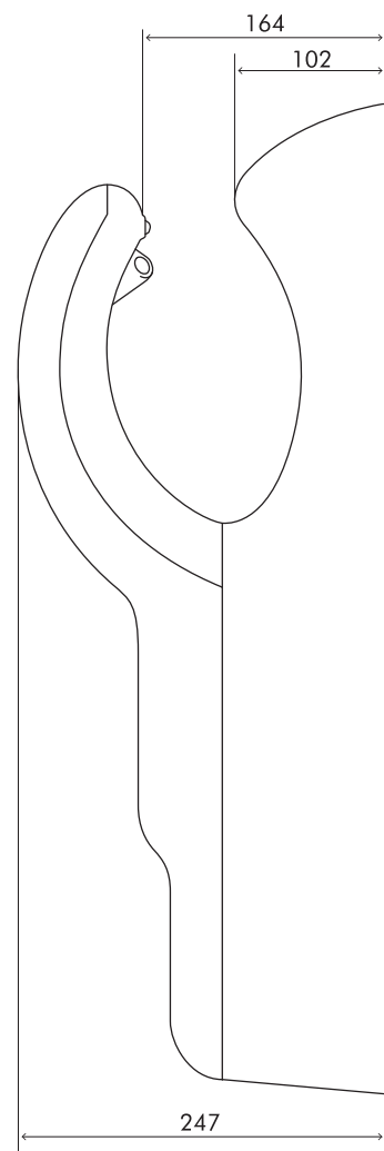
BOČNI PRIKAZ
