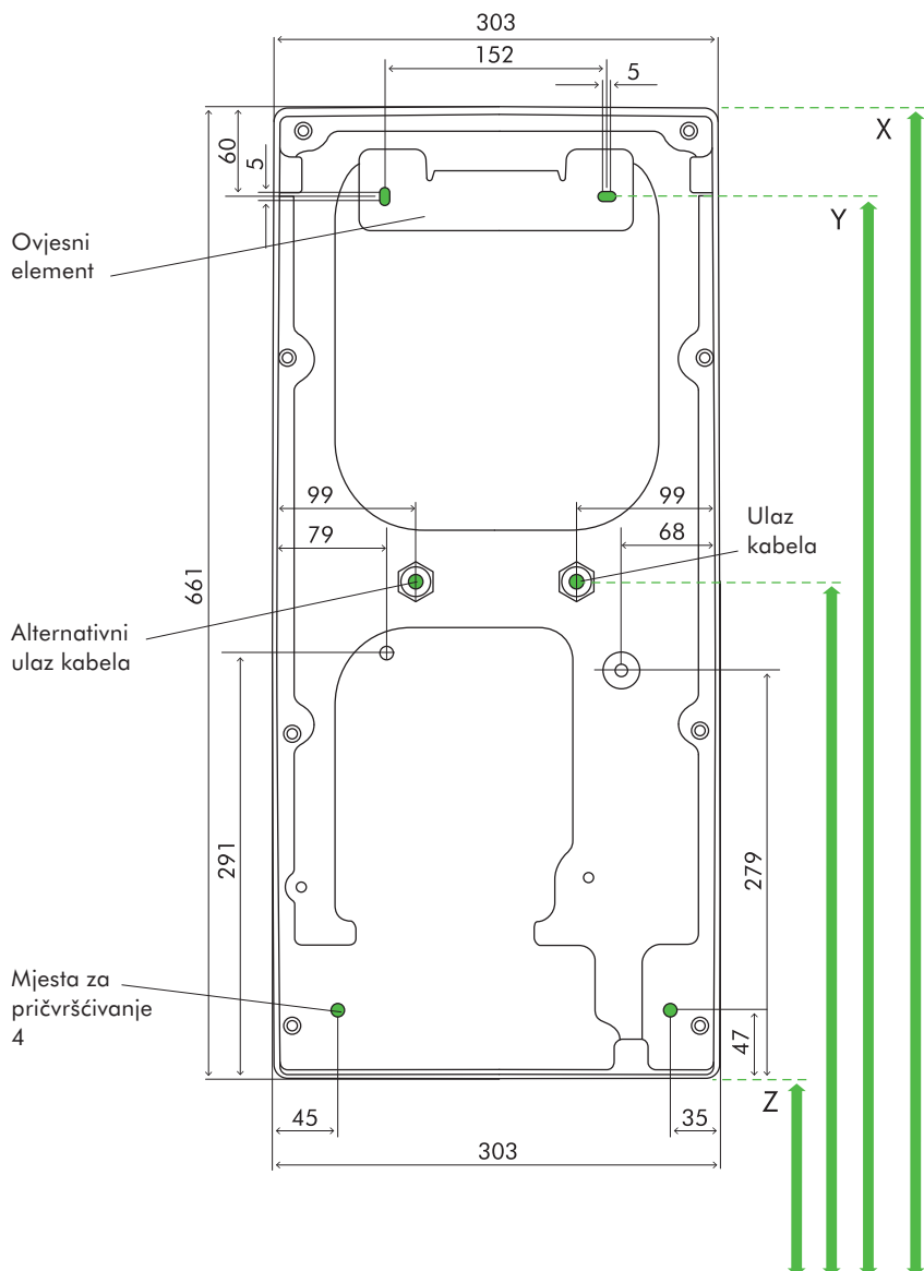
STRAŽNJI PRIKAZ
